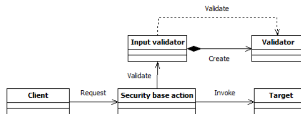
Figure 2 : Patron de sécurité « InterceptingValidator »
